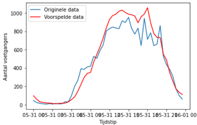
VOORSPELLING SARIMA(0,1,1)(1,1,1)48 MODEL UTRECHT CENTRAAL STATIONSHAL
